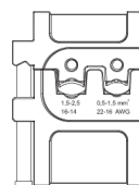
DIE PROFILE
