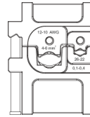
DIE PROFILE
