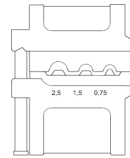
DIE PROFILE
